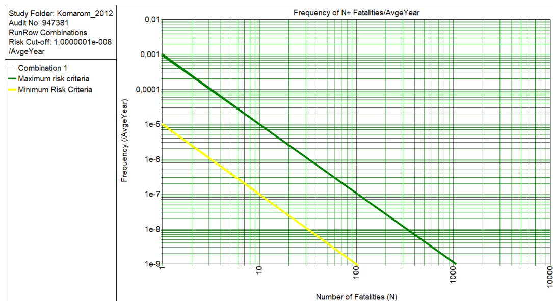
2. ábra: A társadalmi kockázat görbéje (F-N görbe, kék) és a maximális (zöld) ill. a minimális (sárga) kockázati kritérium vonalai.
